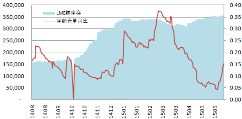
图 4: LME 库存小幅减低, 注销仓单占比上升至 15.1%
